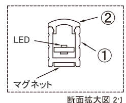
断面拡大図 2:1
